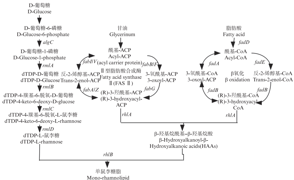
图4 铜绿假单胞菌 A39-1 中鼠李糖脂的合成途径预测
