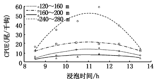
图 4 120 ~ 160 m、160 ~ 200 m、200 ~ 240 m 和 240 ~ 280 m 水层中长鳍金枪鱼渔获率与浸泡时间的关系
