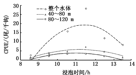
图 3 整个水体、40 ~ 80 m 和 80 ~ 120 m 水层中长鳍金枪鱼渔获率与浸泡时间的关系
